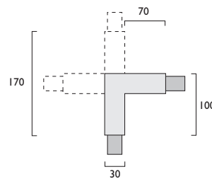
TD1245 A DAT 016 T Inner Connector
