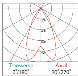
457-458 DLOR: 0.86
