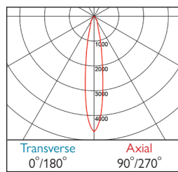
455-456 DLOR: 0.83
