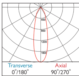
453-454 DLOR: 0.81
